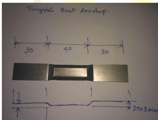
Tungsten Boat
